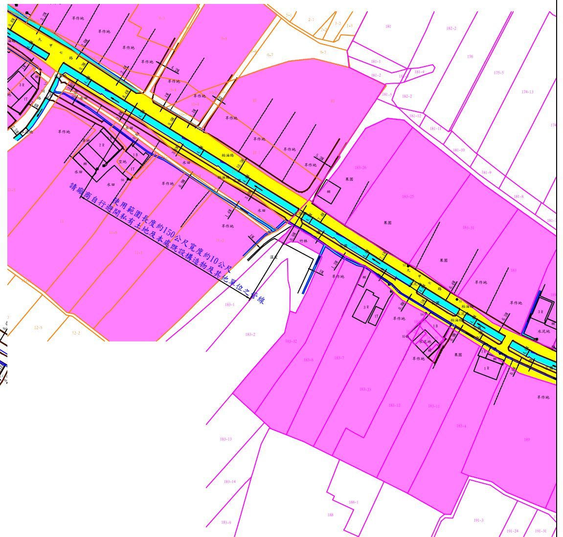
后里圳后里區月眉段473地號小水力發電設備建置現地平面圖
