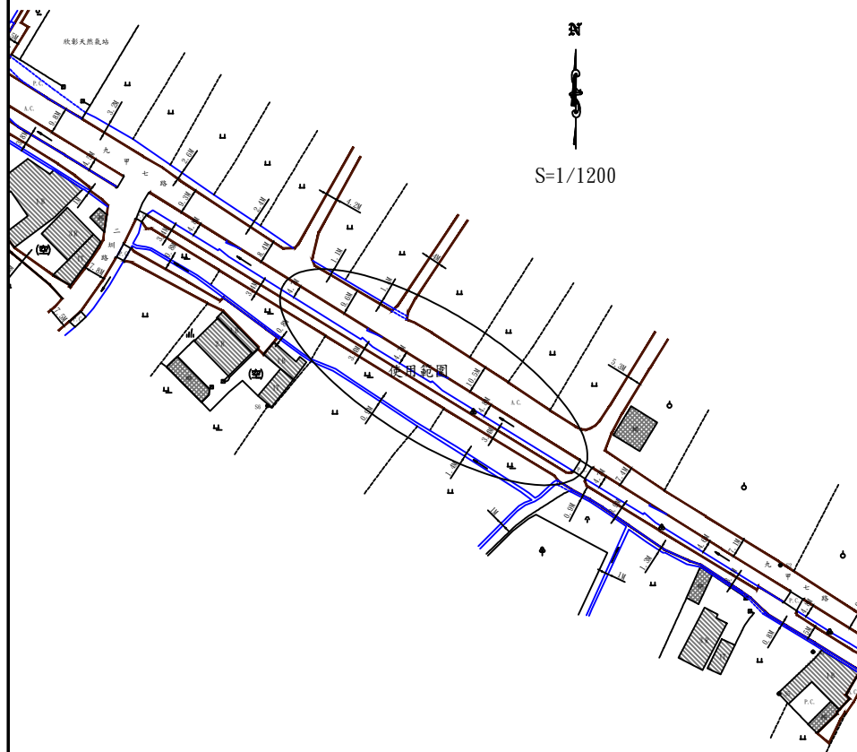
后里圳后里區月眉段473地號小水力發電設備建置現地平面圖
